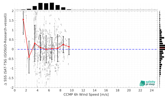
(d) CCMP Wind Speed
