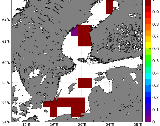
(f) STD( \Delta SSS) (Satellite - Argo)
