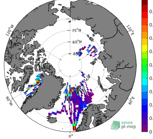
(d) Std(TSG-POLARSTERN SSS)
