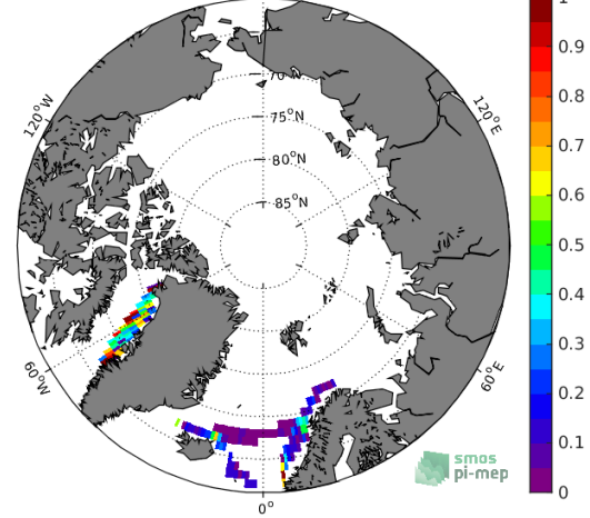
(d) Std(TSG-LEGOS-DM SSS)
