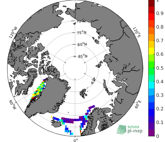
(f) Std( \Delta SSS) (Satellite - TSG-LEGOS-DM)
