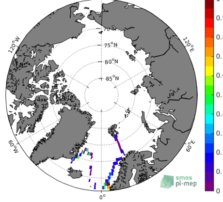
(d) Std(TSG-GOSUD-Research-vessel SSS)
