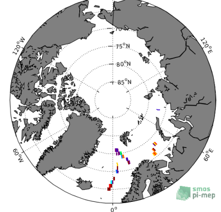
(f) Std( \Delta SSS) (Satellite - TSG-GOSUD-Sailing-ship)
