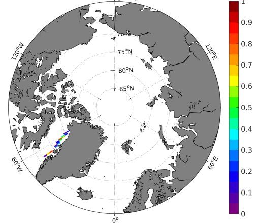
(f) STD( \Delta SSS) (Satellite - TSG-GOSUD-Sailing-ship)
