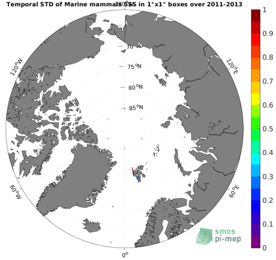
(d) Std(Marine mammals SSS)
