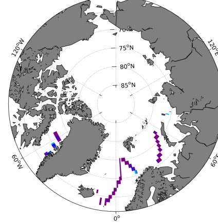
(f) STD( \Delta SSS) (Satellite - TSG-GOSUD-Sailing-ship)
