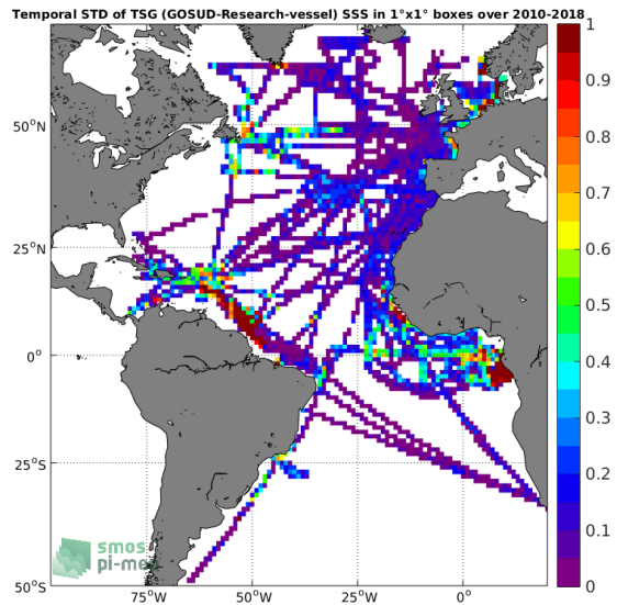
(d) Std(TSG (GOSUD-Research-vessel) SSS)
