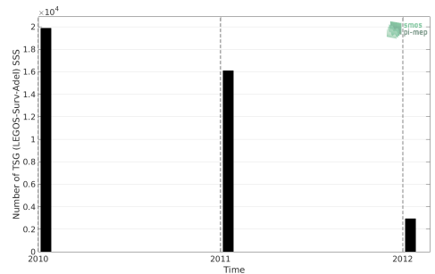
(h) TSG (LEGOS-Survostral-Adélie)
