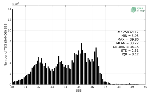
(d) TSG (SAMOS)
