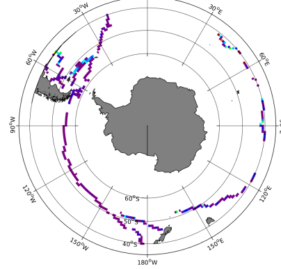
(d) STD(TSG-GOSUD-Sailing-ship SSS)
