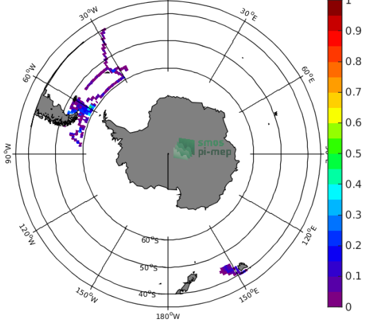
(b) Std(Satellite SSS)
