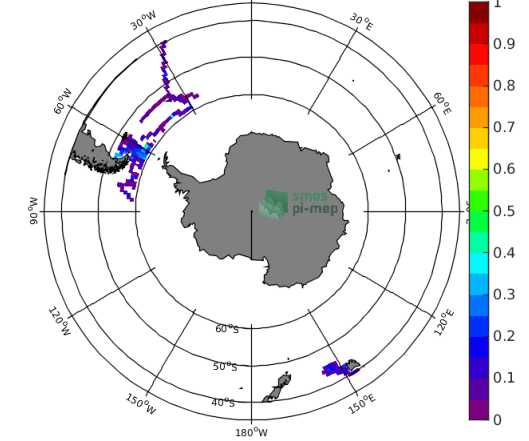
(f) Std( \Delta SSS) (Satellite - TSG-SAMOS)
