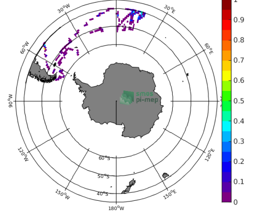
(d) Std(TSG-POLARSTERN SSS)
