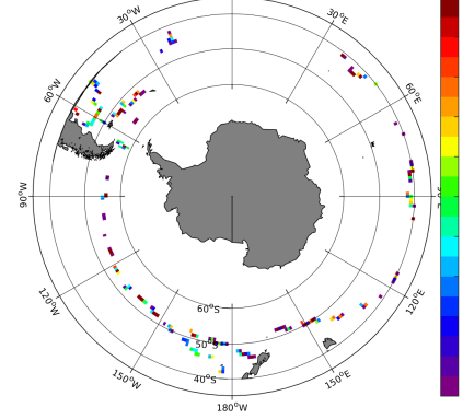
(f) STD( \Delta SSS) (Satellite - TSG-GOSUD-Sailing-ship)
