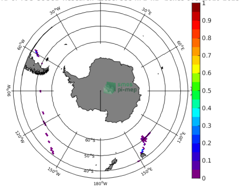
(d) Std(TSG-GOSUD-Research-vessel SSS)
