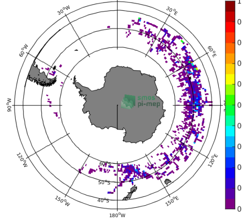
(d) Std(Sea mammals SSS)
