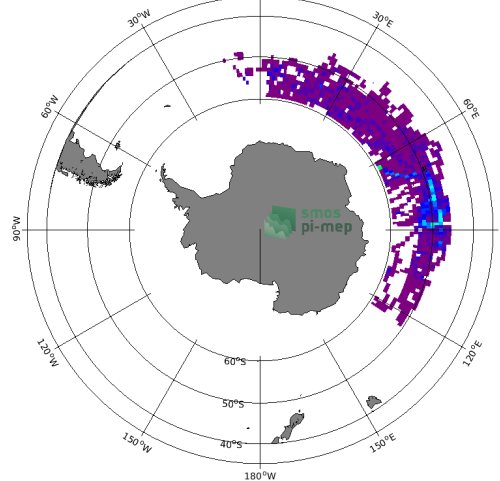
(d) Std(Sea mammals SSS)
