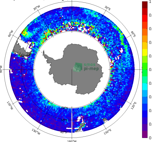
(f) Std( \Delta SSS) (Satellite - Argo)
