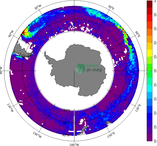
(d) Std(Argo SSS)
