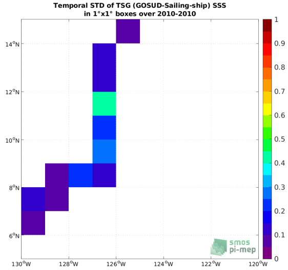
(d) Std(TSG (GOSUD-Sailing-ship) SSS)
