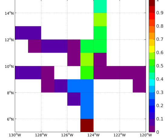
(d) STD(TSG-SAMOS SSS)
